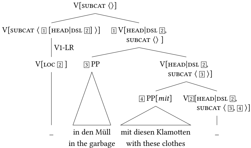
Figure 21.22: HPSG variant of the analysis of In den Müll mit diesen Klamotten!/?
