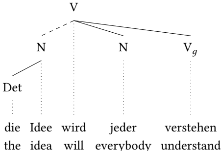
Figure 20.5: Analysis of Die Idee wird jeder verstehen . ‘Everybody will understand the idea.’ involving rising
